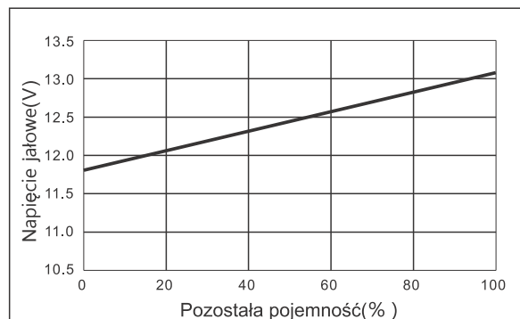
Krzywa napięcia jałowego vs. pojemność
