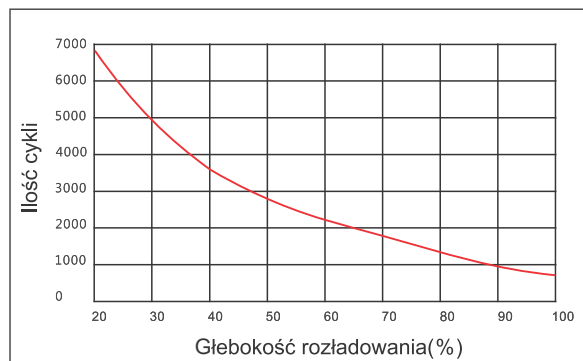
Wpływ głębokości rozł. na pracę cykliczną
