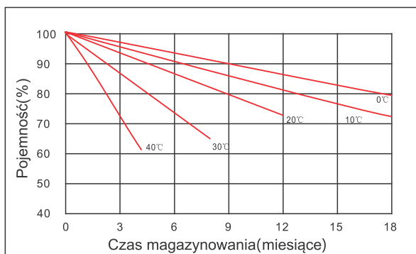
Krzywe samorozładowania
