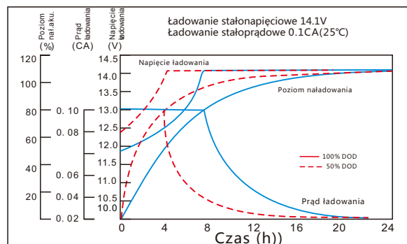
Charakterystyka ładowania
